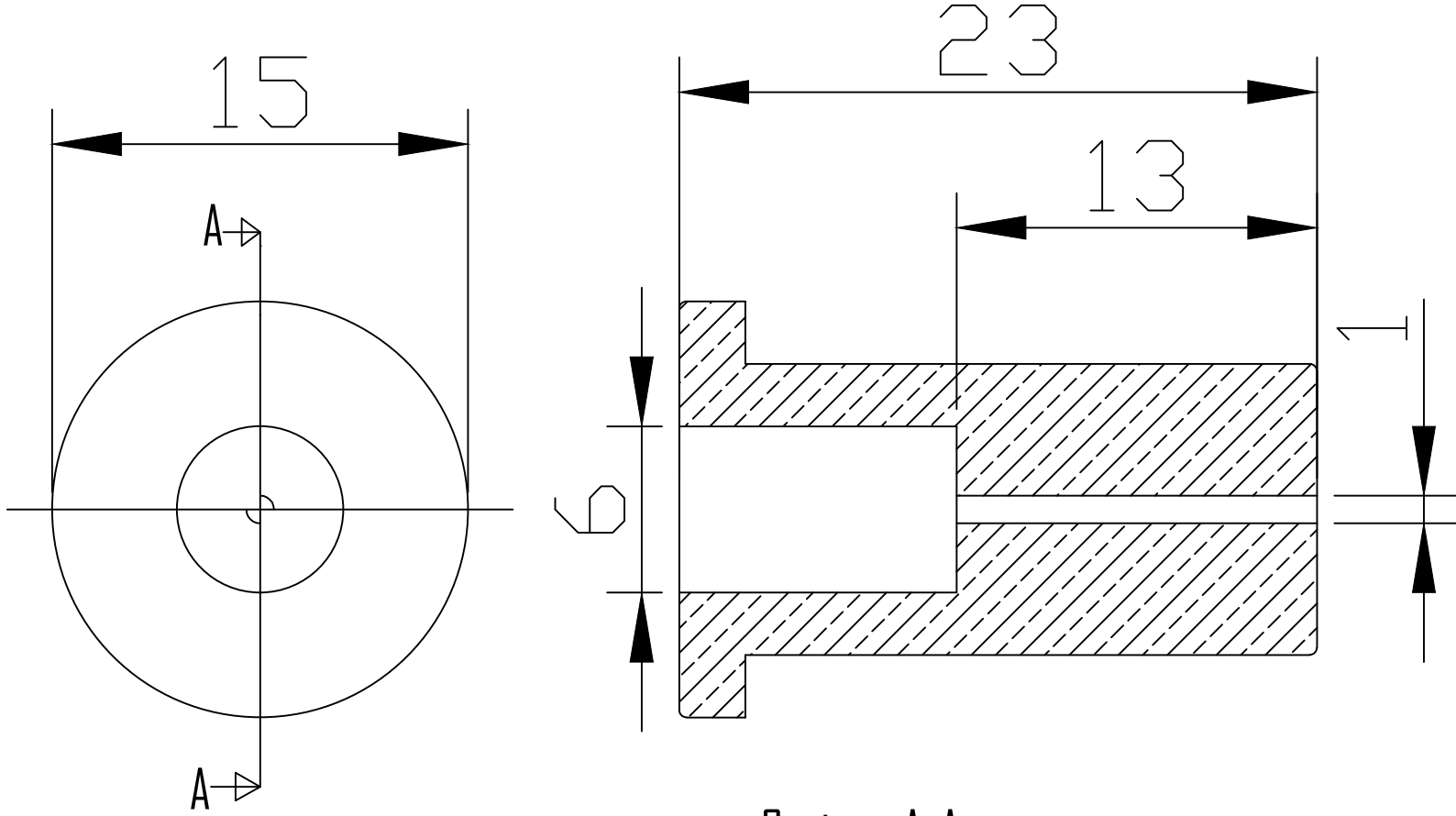
Sezione A-A
